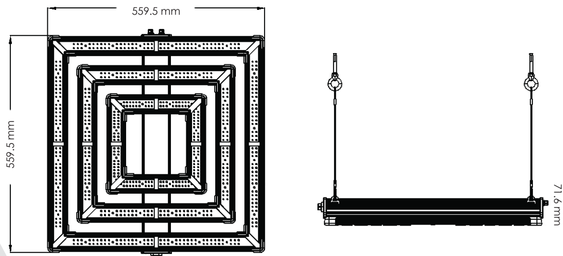
Fig 1. Dimensioni dell'apparecchio
