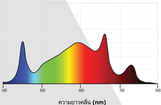
รูปที่สอง กราฟ SQR แสดงเต็มสเปกตรัม +
